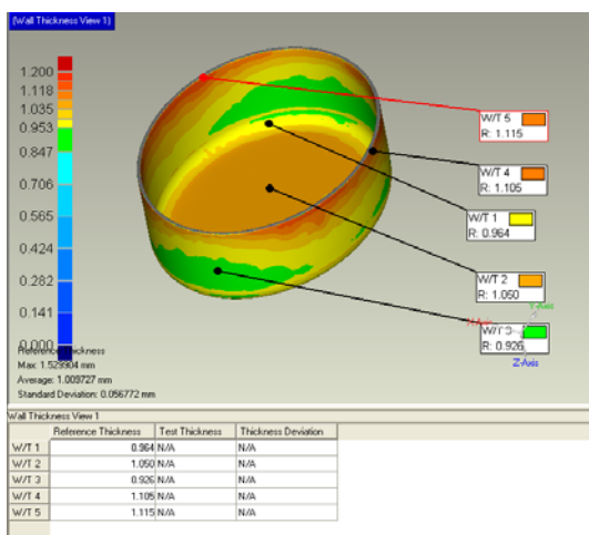
Slika 5. Raspodjela debljine po izvučenom tijelu elipsastog presjeka
